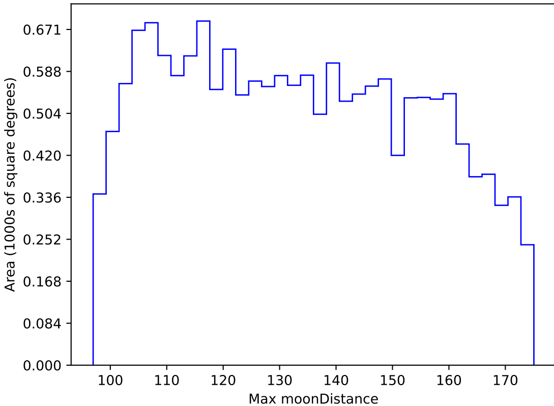
retro_baseline_v2.0_10yrs WFD y band: Max moonDistance
