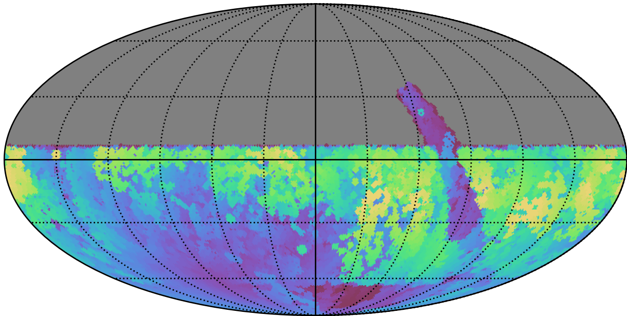
retro_baseline_v2.0_10yrs All sky y band: Max moonDistance
