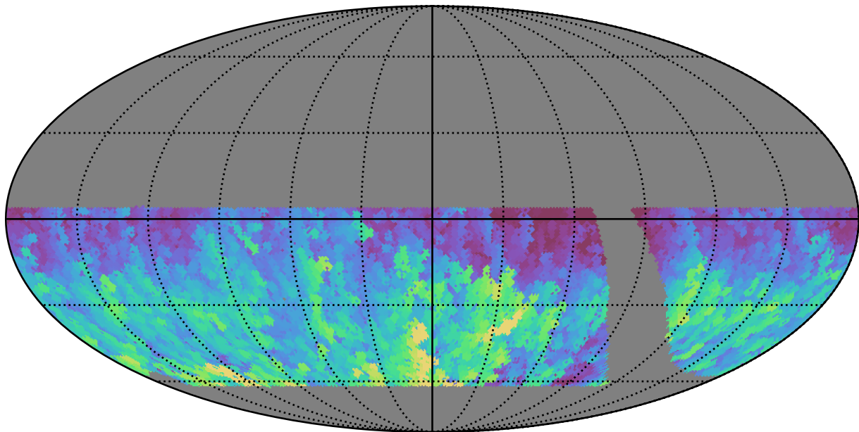
retro_baseline_v2.0_10yrs WFD z band: Max HA
