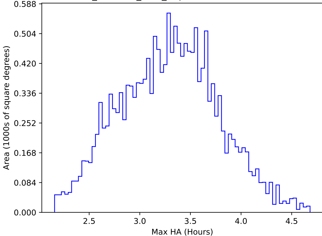
retro_baseline_v2.0_10yrs WFD z band: Max HA
