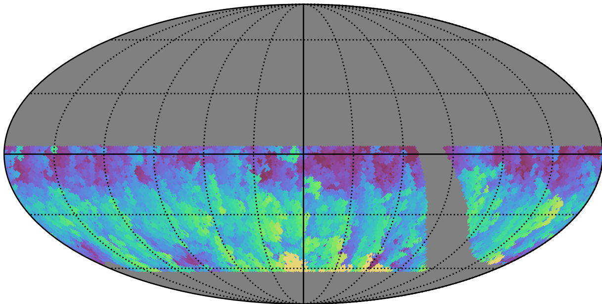
retro_baseline_v2.0_10yrs WFD u band: Max HA
