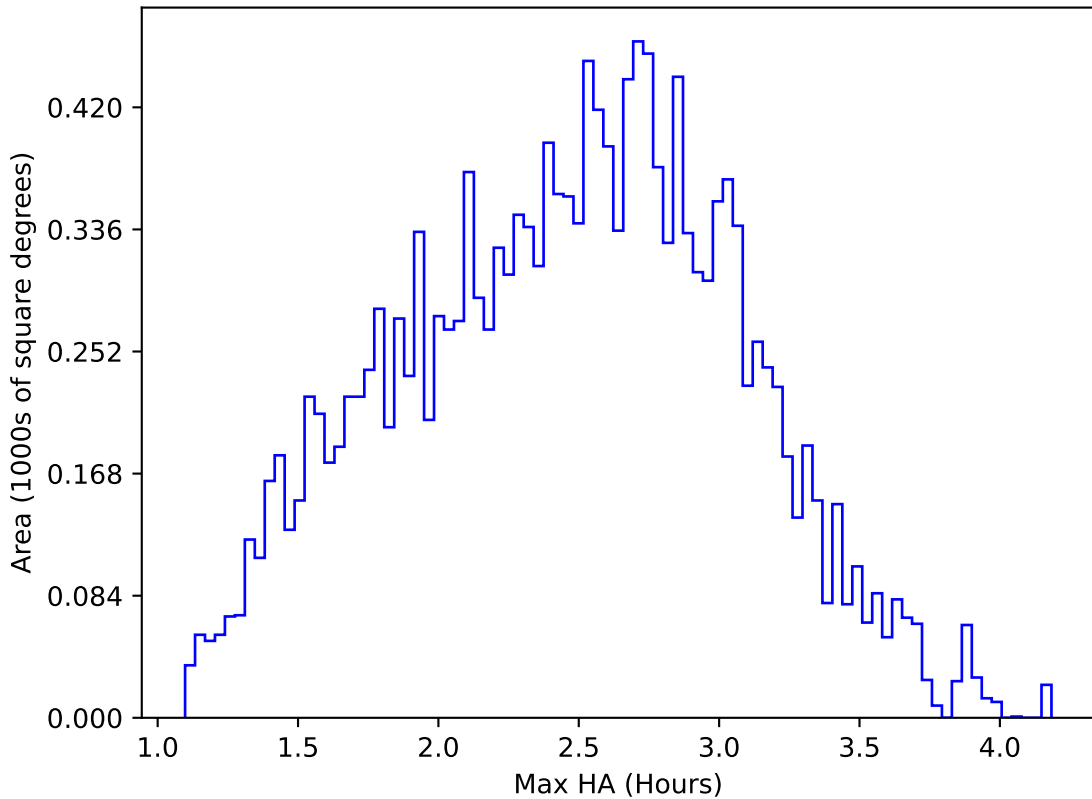
retro_baseline_v2.0_10yrs WFD u band: Max HA
