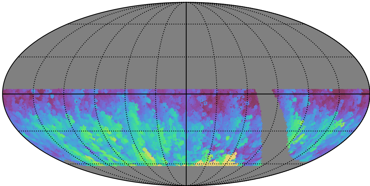
retro_baseline_v2.0_10yrs WFD r band: Max HA
