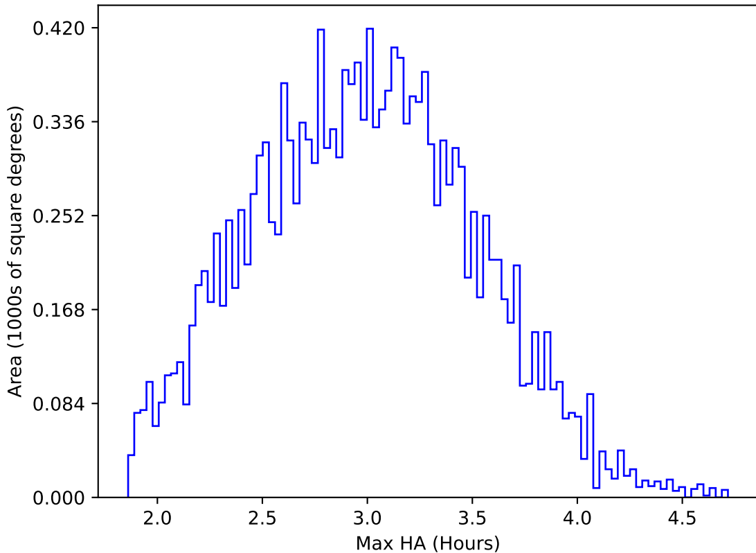
retro_baseline_v2.0_10yrs WFD r band: Max HA
