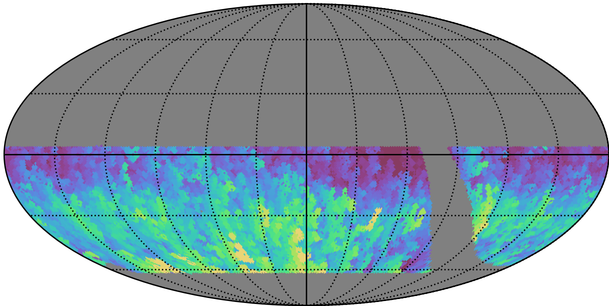
retro_baseline_v2.0_10yrs WFD i band: Max HA
