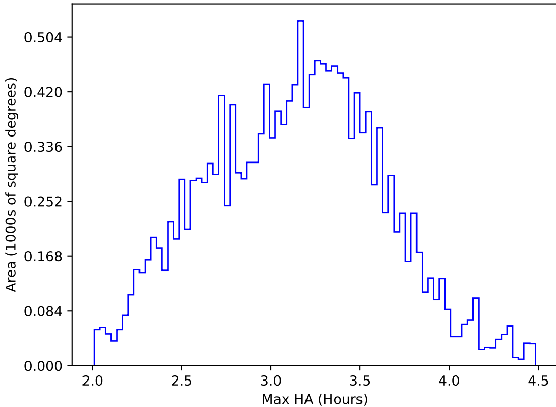
retro_baseline_v2.0_10yrs WFD i band: Max HA
