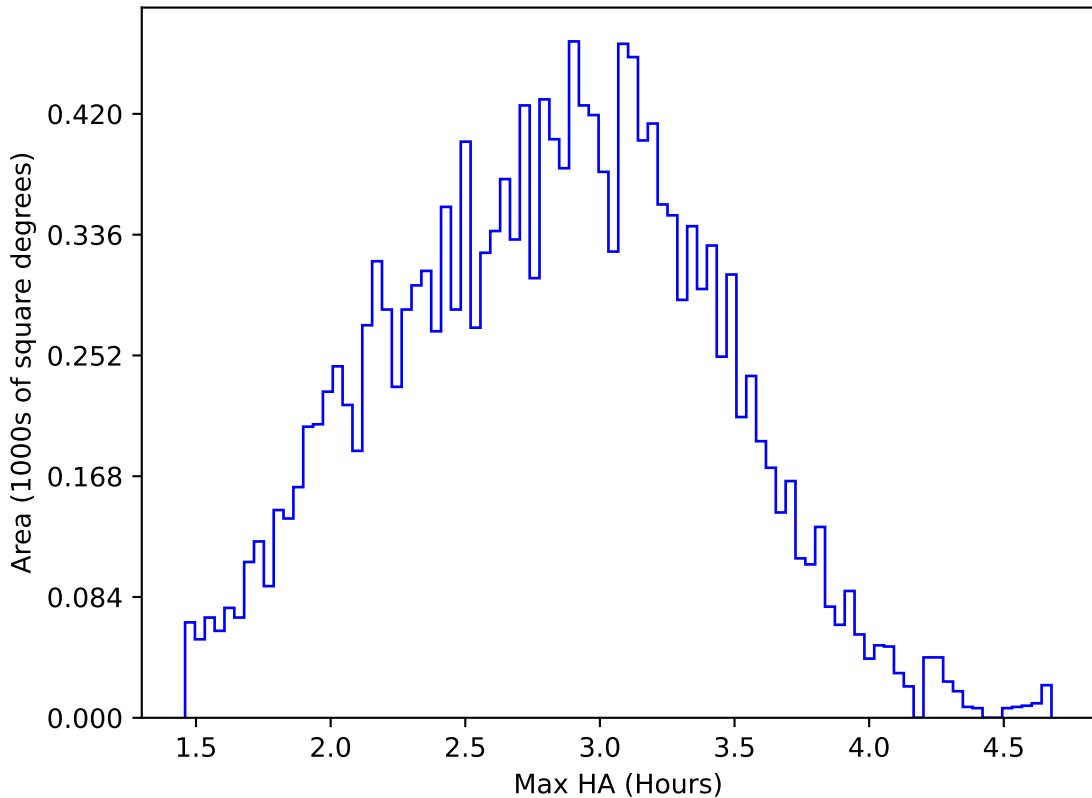
retro_baseline_v2.0_10yrs WFD g band: Max HA
