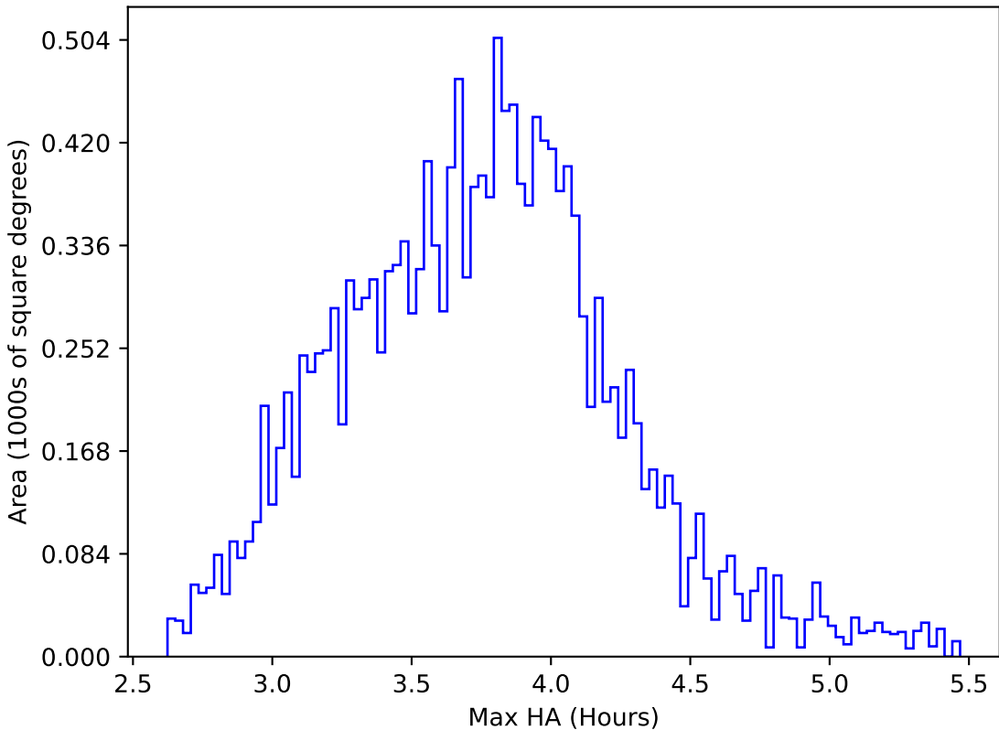
retro_baseline_v2.0_10yrs WFD all bands: Max HA
