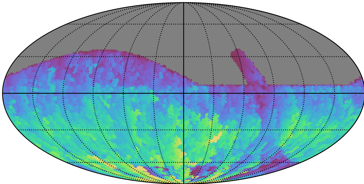
retro_baseline_v2.0_10yrs All sky z band: Max HA
