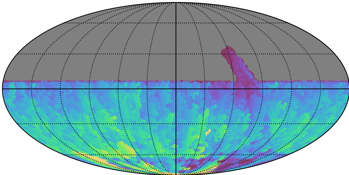
retro_baseline_v2.0_10yrs All sky y band: Max HA
