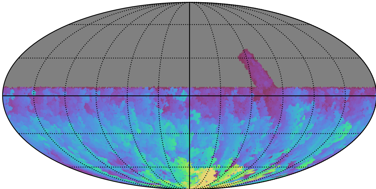
retro_baseline_v2.0_10yrs All sky u band: Max HA
