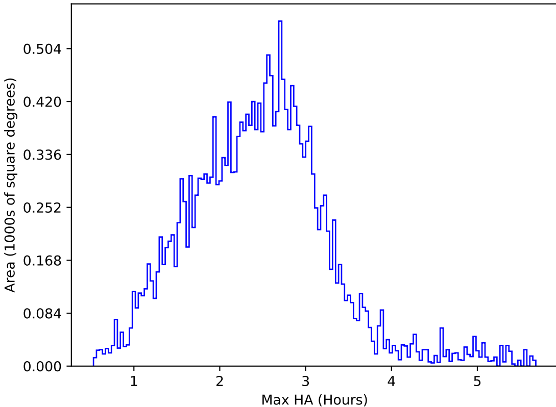
retro_baseline_v2.0_10yrs All sky u band: Max HA
