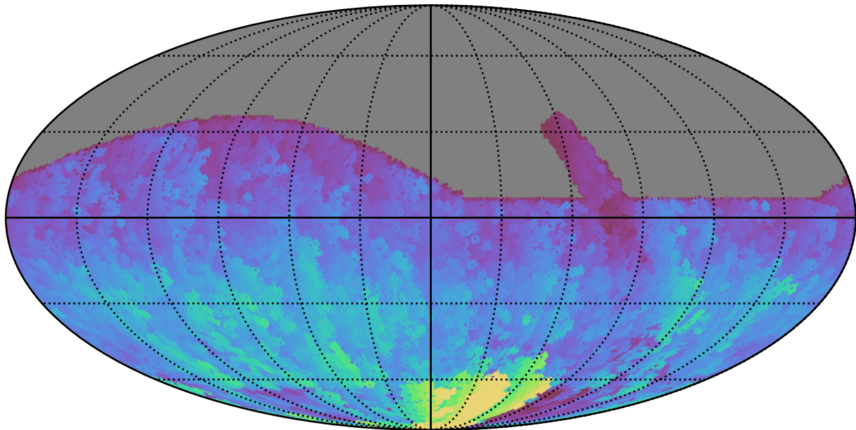
retro_baseline_v2.0_10yrs All sky r band: Max HA
