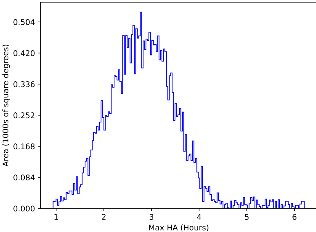
retro_baseline_v2.0_10yrs All sky r band: Max HA
