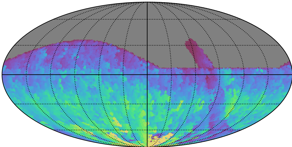
retro_baseline_v2.0_10yrs All sky i band: Max HA
