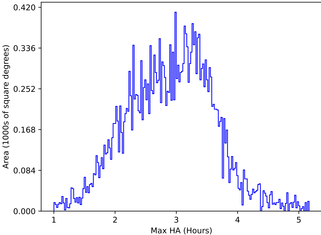
retro_baseline_v2.0_10yrs All sky i band: Max HA
