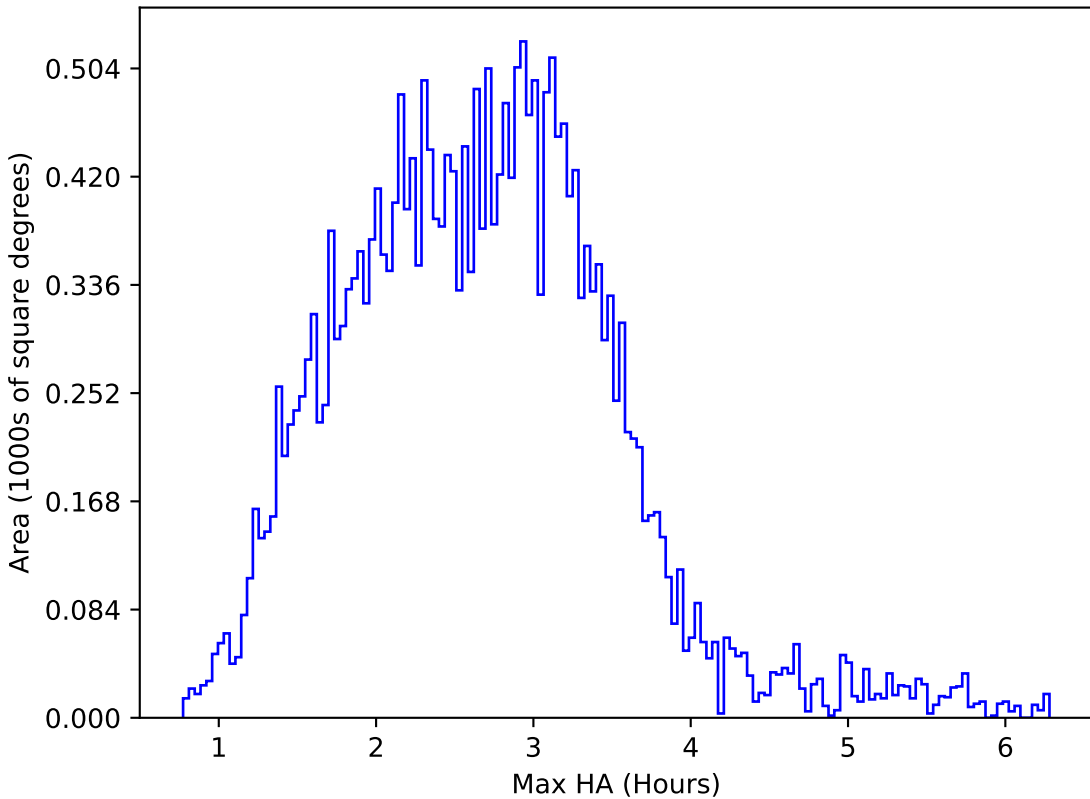
retro_baseline_v2.0_10yrs All sky g band: Max HA
