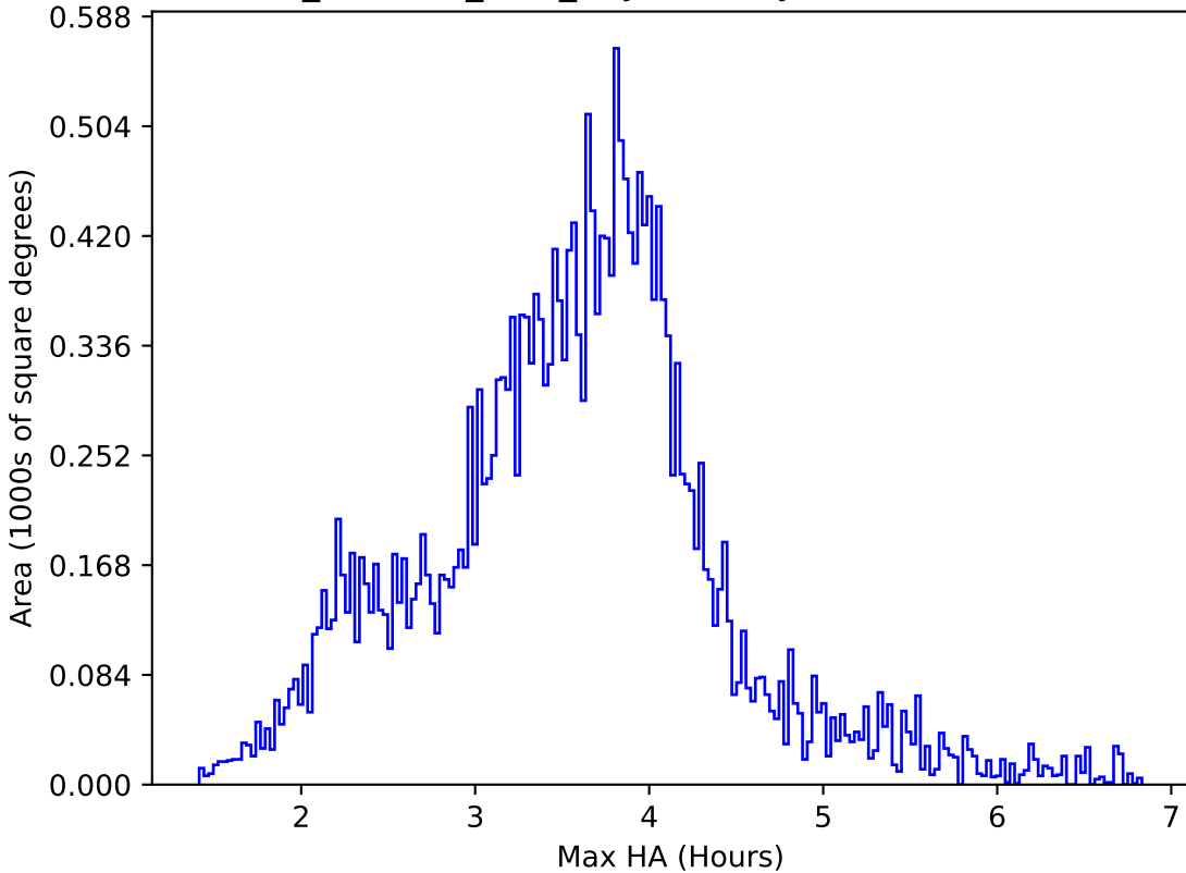
retro_baseline_v2.0_10yrs All sky all bands: Max HA
