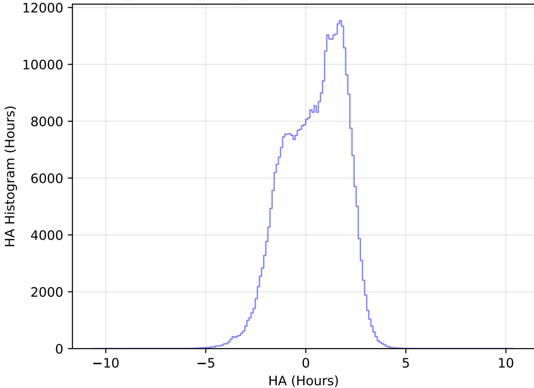
retro_baseline_v2.0_10yrs All sky z band: HA Histogram
