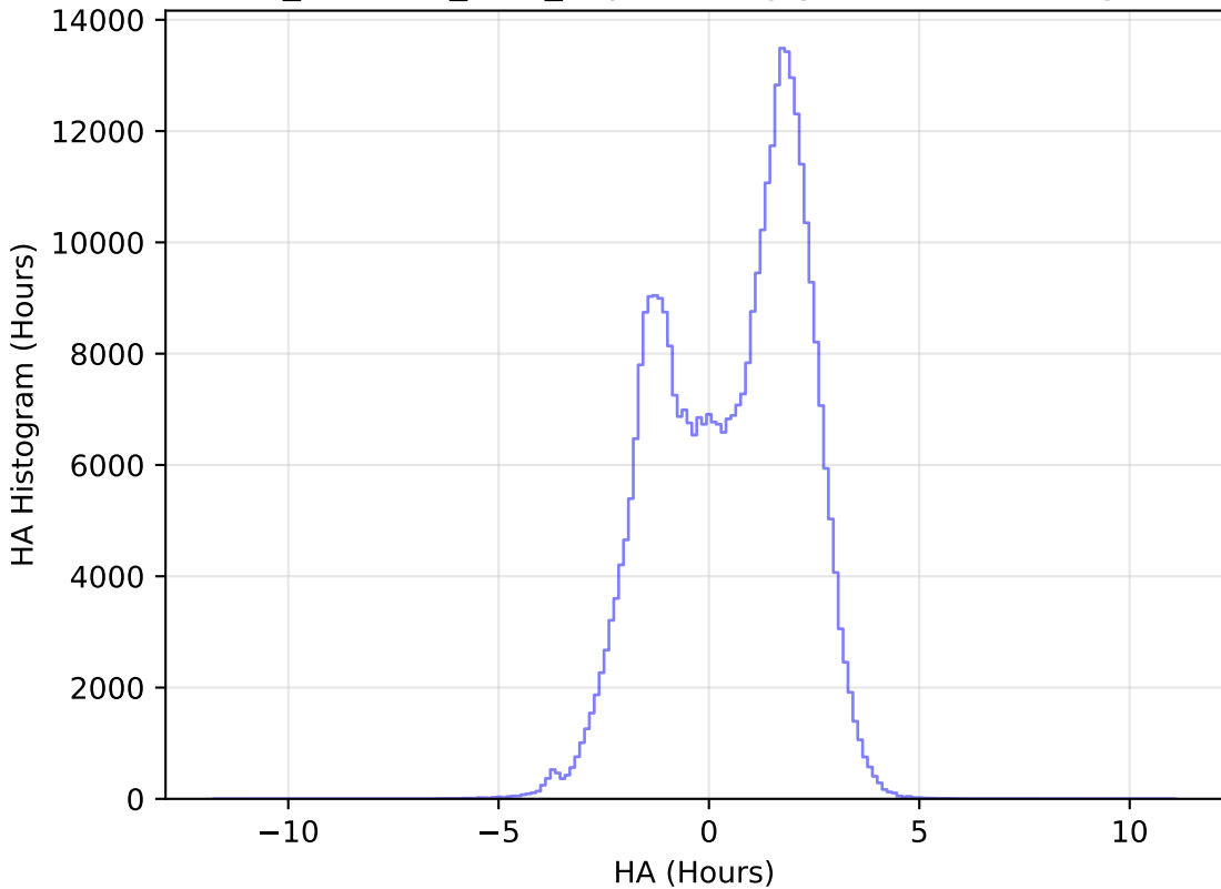
retro_baseline_v2.0_10yrs All sky y band: HA Histogram
