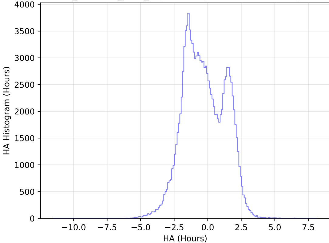
retro_baseline_v2.0_10yrs All sky u band: HA Histogram
