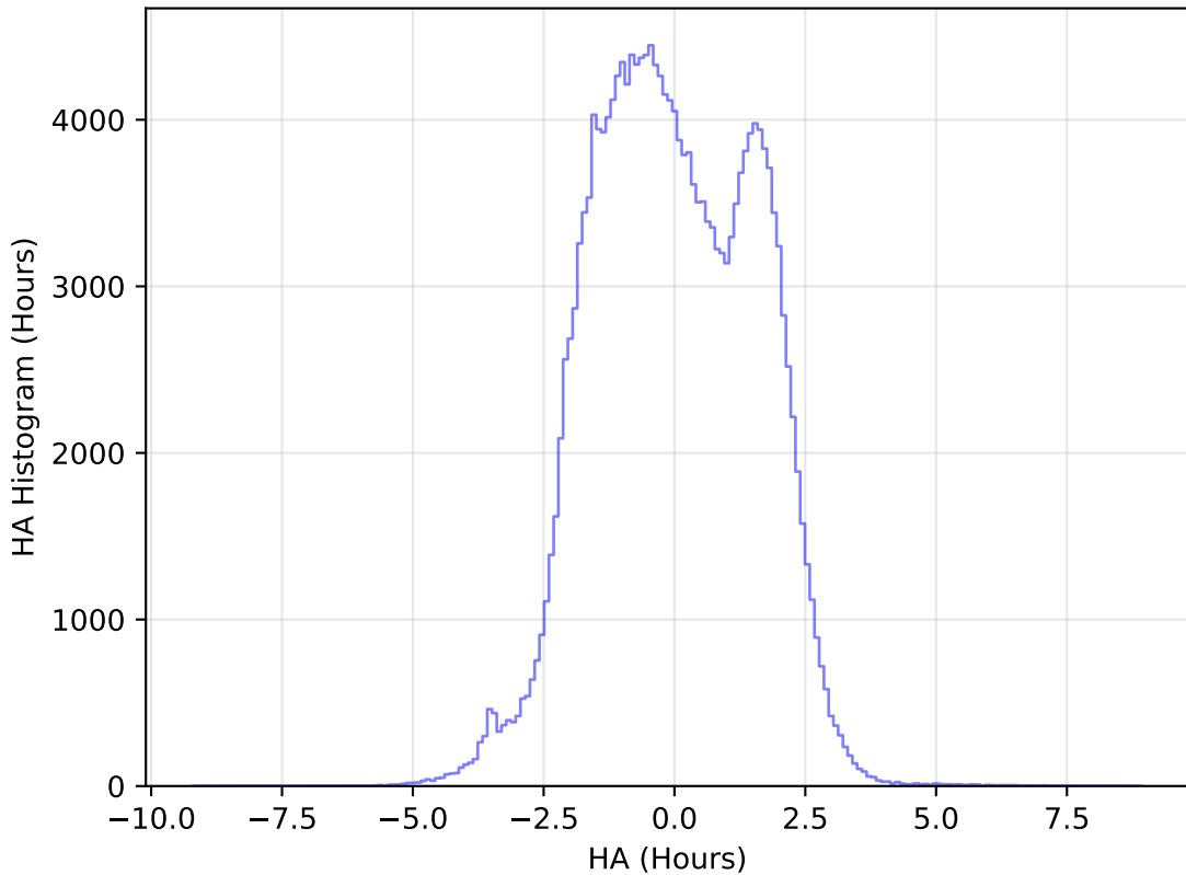
retro_baseline_v2.0_10yrs All sky g band: HA Histogram
