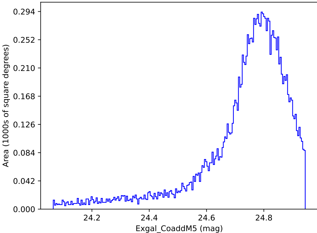
retro_baseline_v2.0_10yrs WFD y band: Exgal_CoaddM5
