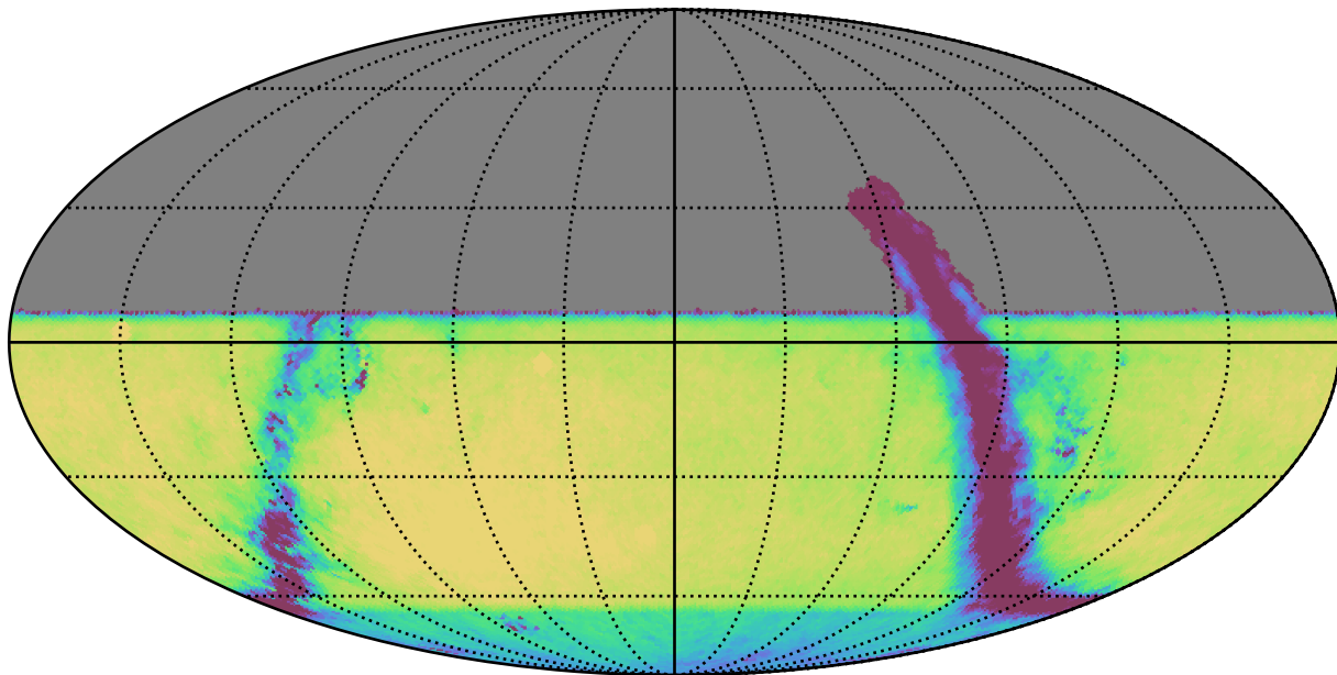
retro_baseline_v2.0_10yrs All sky y band: Exgal_CoaddM5
