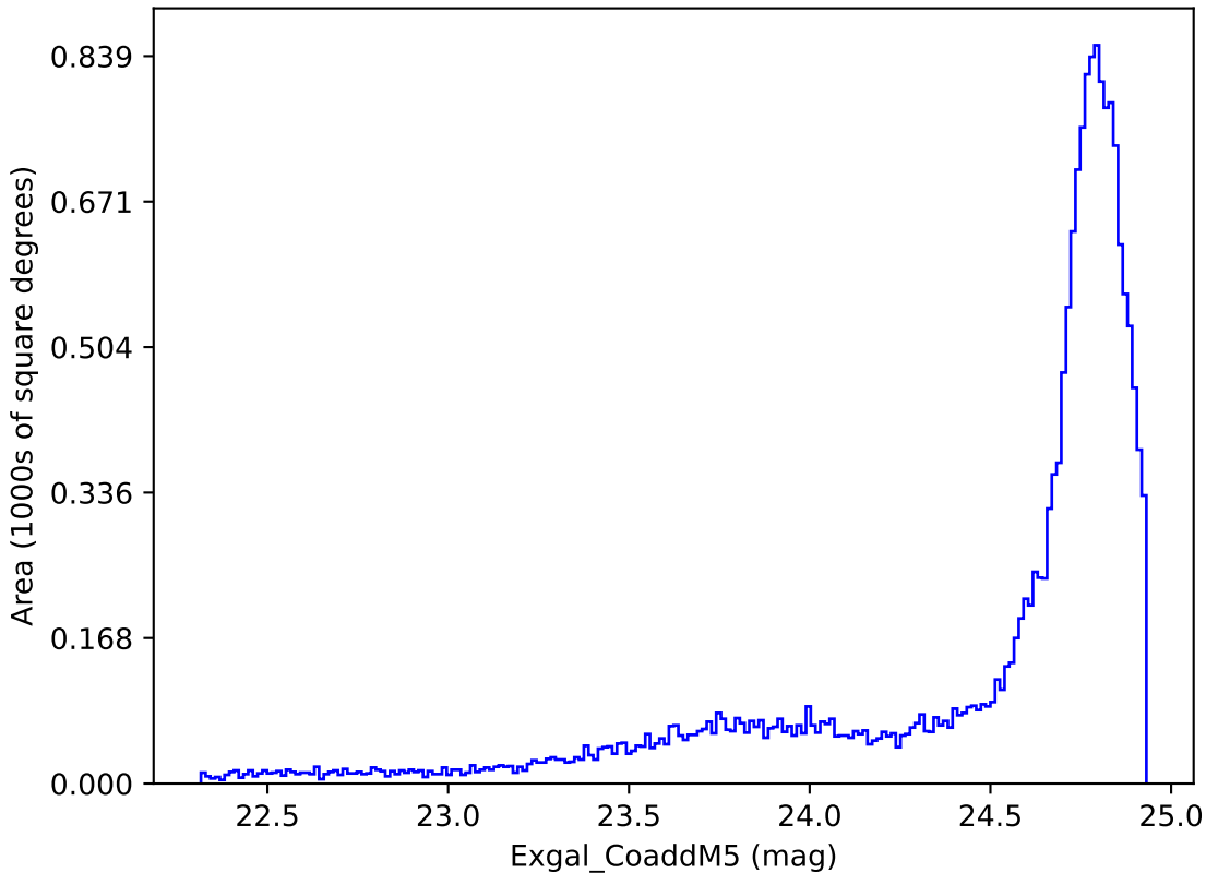
retro_baseline_v2.0_10yrs All sky y band: Exgal_CoaddM5
