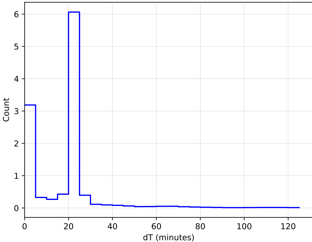
1e6 retro_baseline_v2.0_10yrs WFD: DeltaT Histogram
