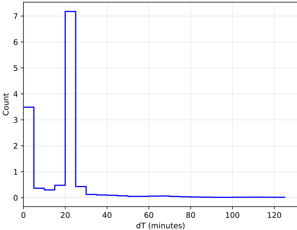
1e6 retro_baseline_v2.0_10yrs All sky: DeltaT Histogram
