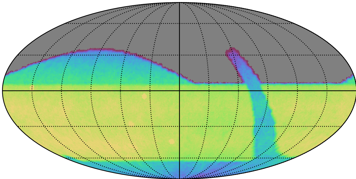
retro_baseline_v2.0_10yrs All sky z band: CoaddM5
