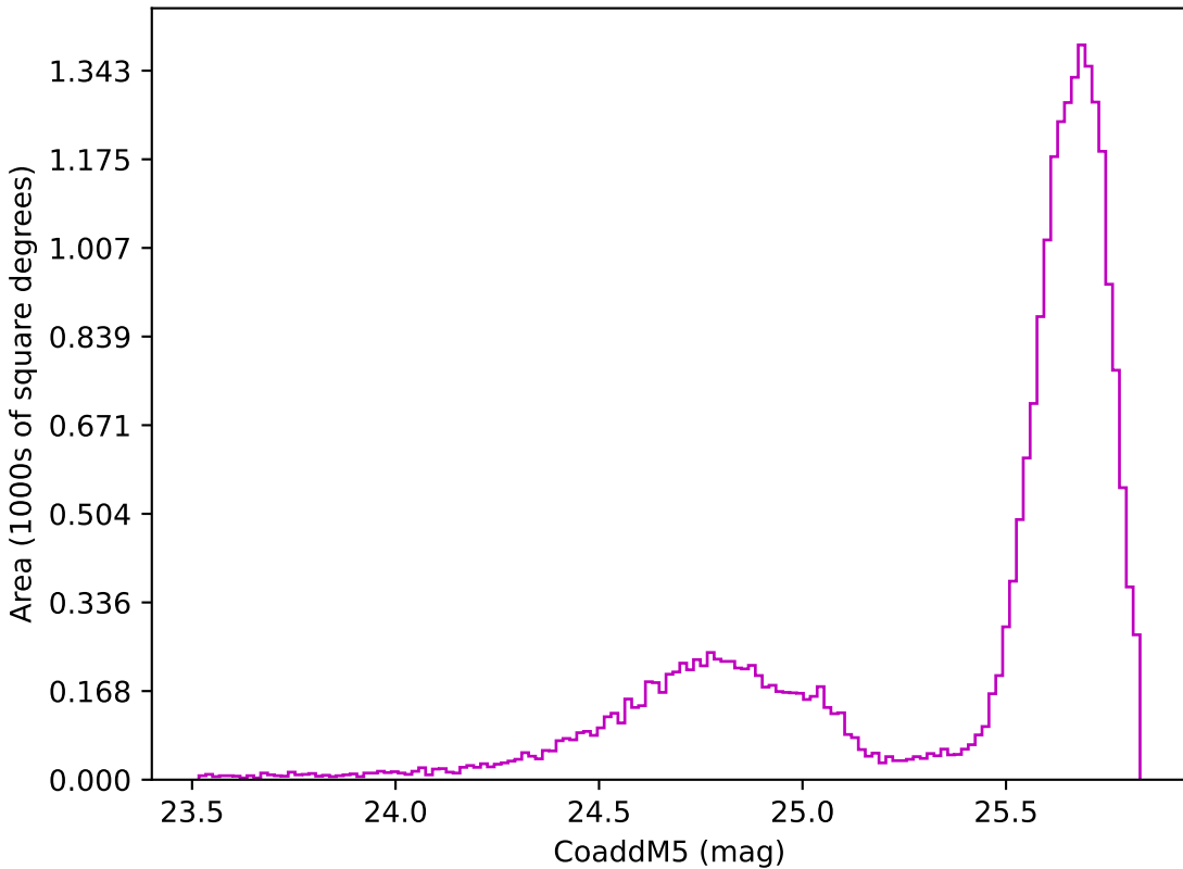
retro_baseline_v2.0_10yrs All sky z band: CoaddM5
