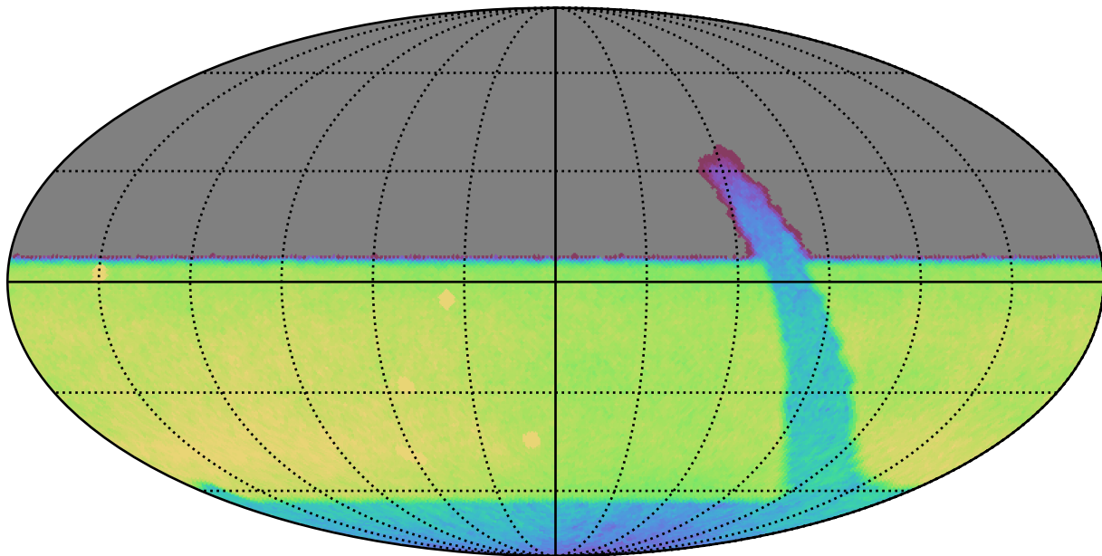
retro_baseline_v2.0_10yrs All sky y band: CoaddM5
