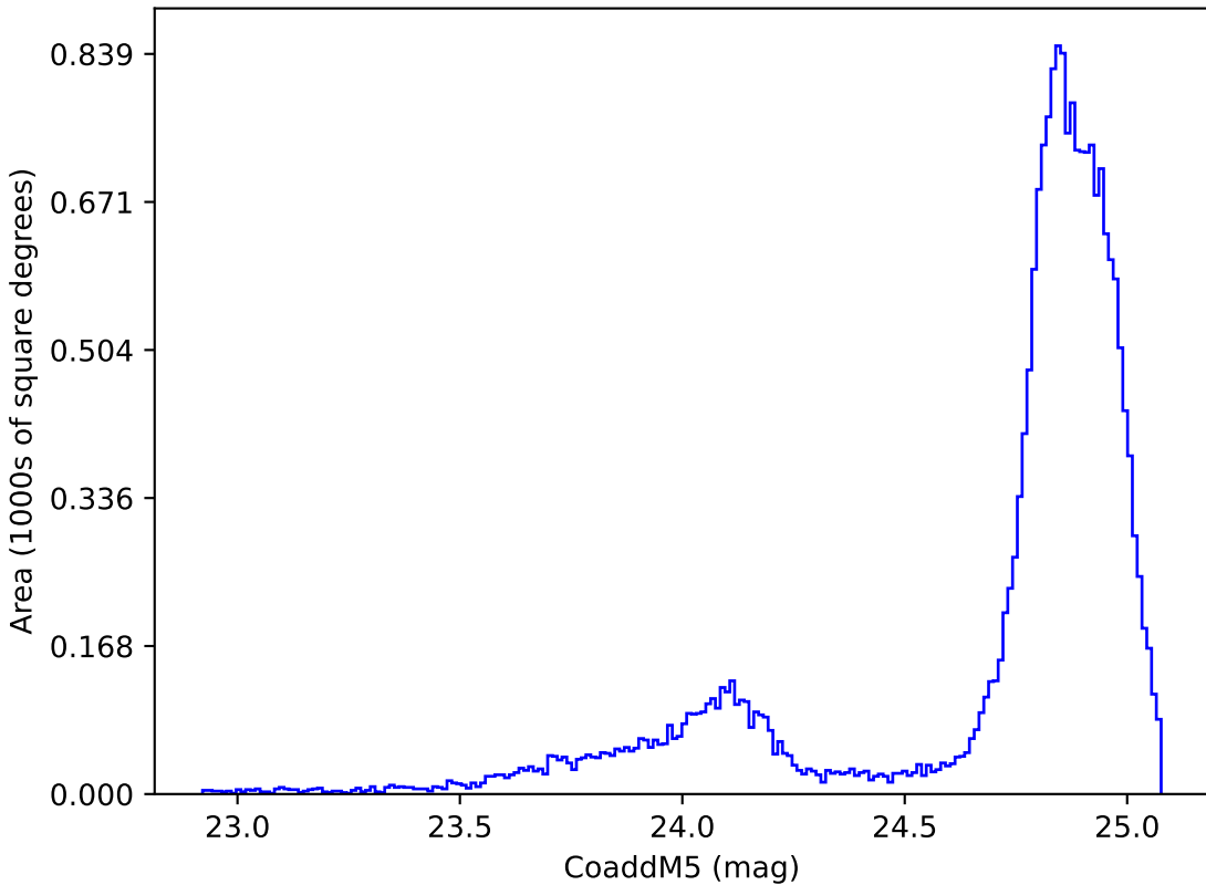
retro_baseline_v2.0_10yrs All sky y band: CoaddM5
