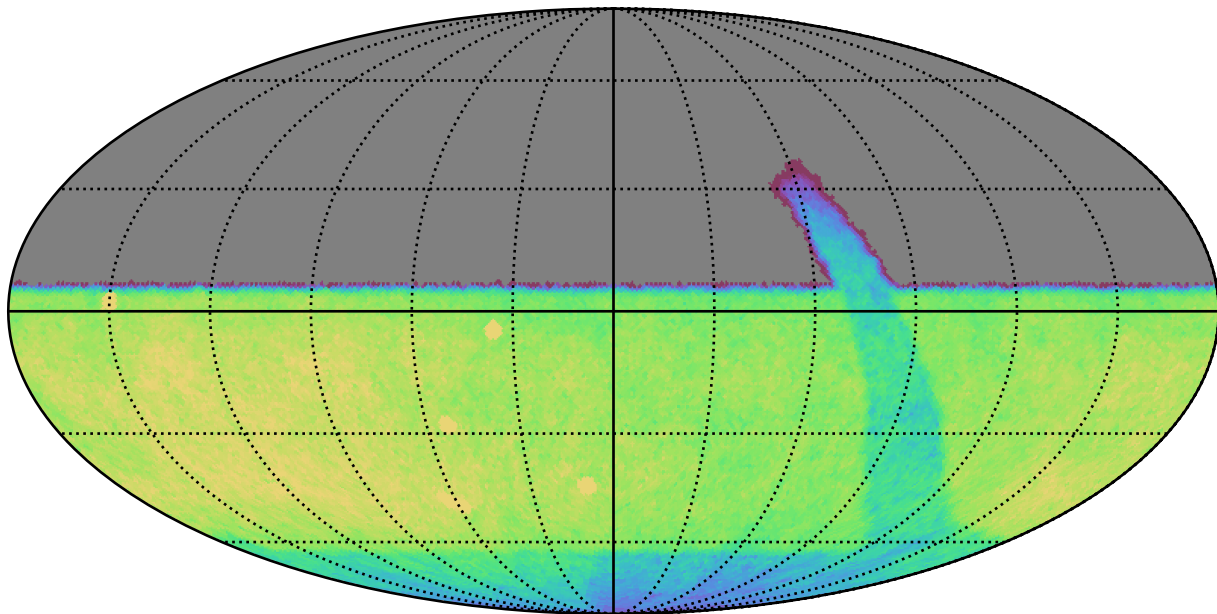
retro_baseline_v2.0_10yrs All sky u band: CoaddM5
