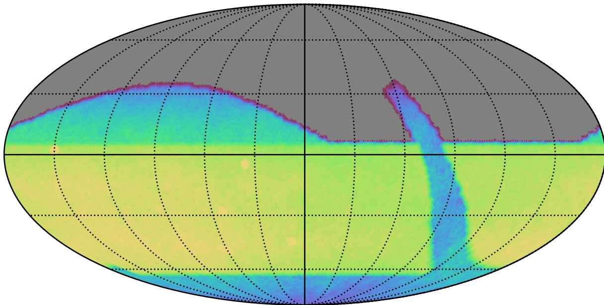
retro_baseline_v2.0_10yrs All sky r band: CoaddM5
