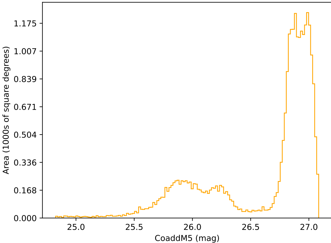
retro_baseline_v2.0_10yrs All sky r band: CoaddM5
