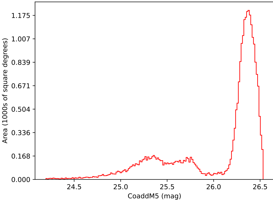
retro_baseline_v2.0_10yrs All sky i band: CoaddM5
