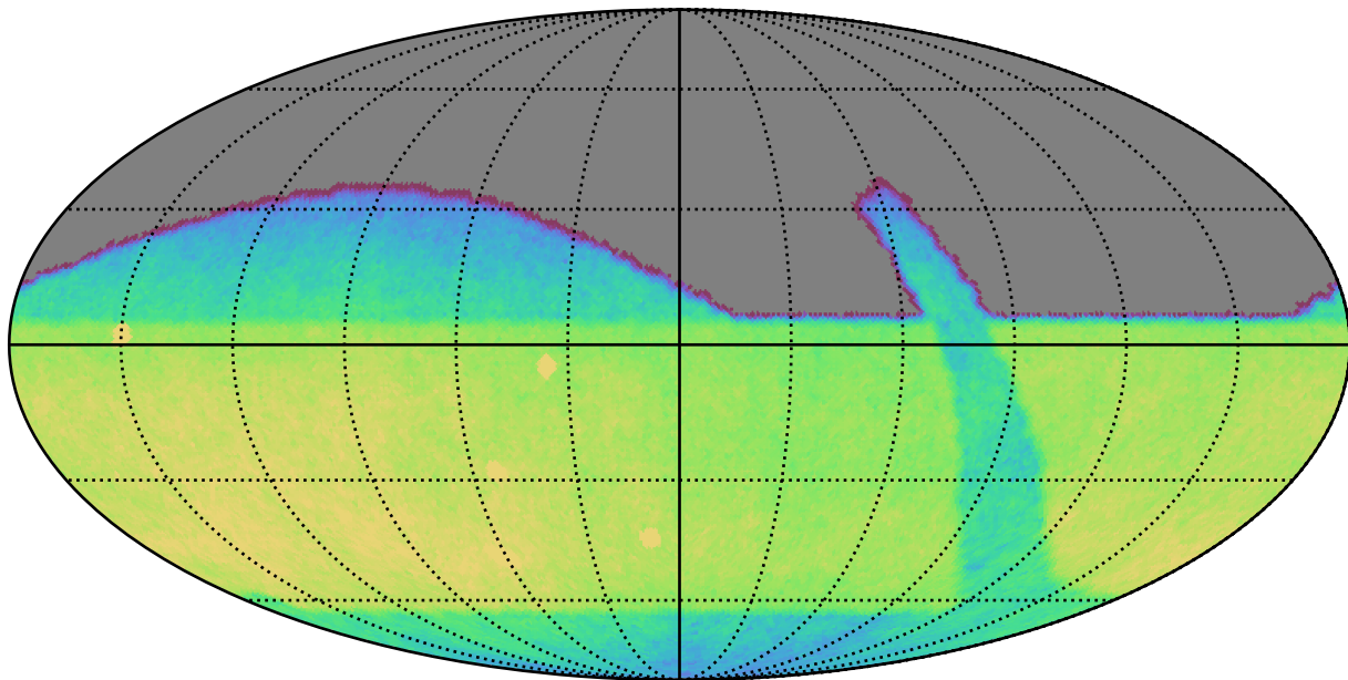
retro_baseline_v2.0_10yrs All sky g band: CoaddM5
