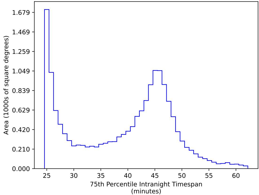
retro_baseline_v2.0_10yrs WFD iz bands: 75th Percentile Intranight Timespan
