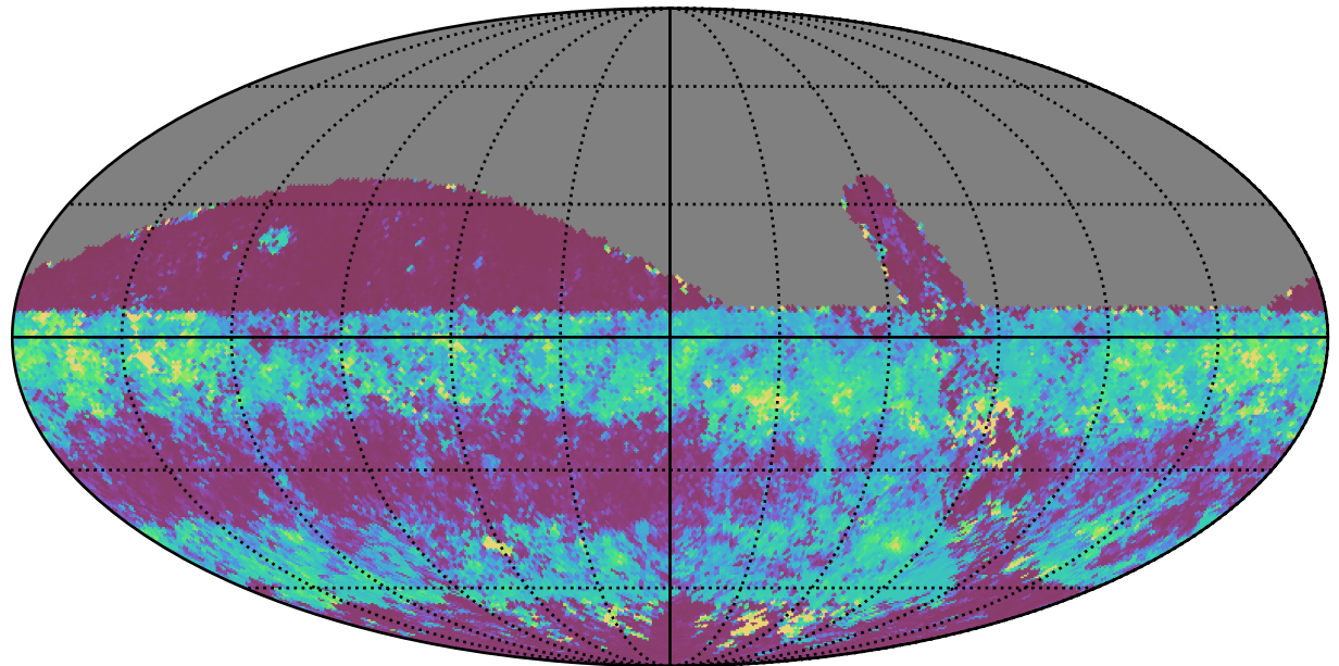
retro_baseline_v2.0_10yrs All sky iz bands: 75th Percentile Intranight Timespan
