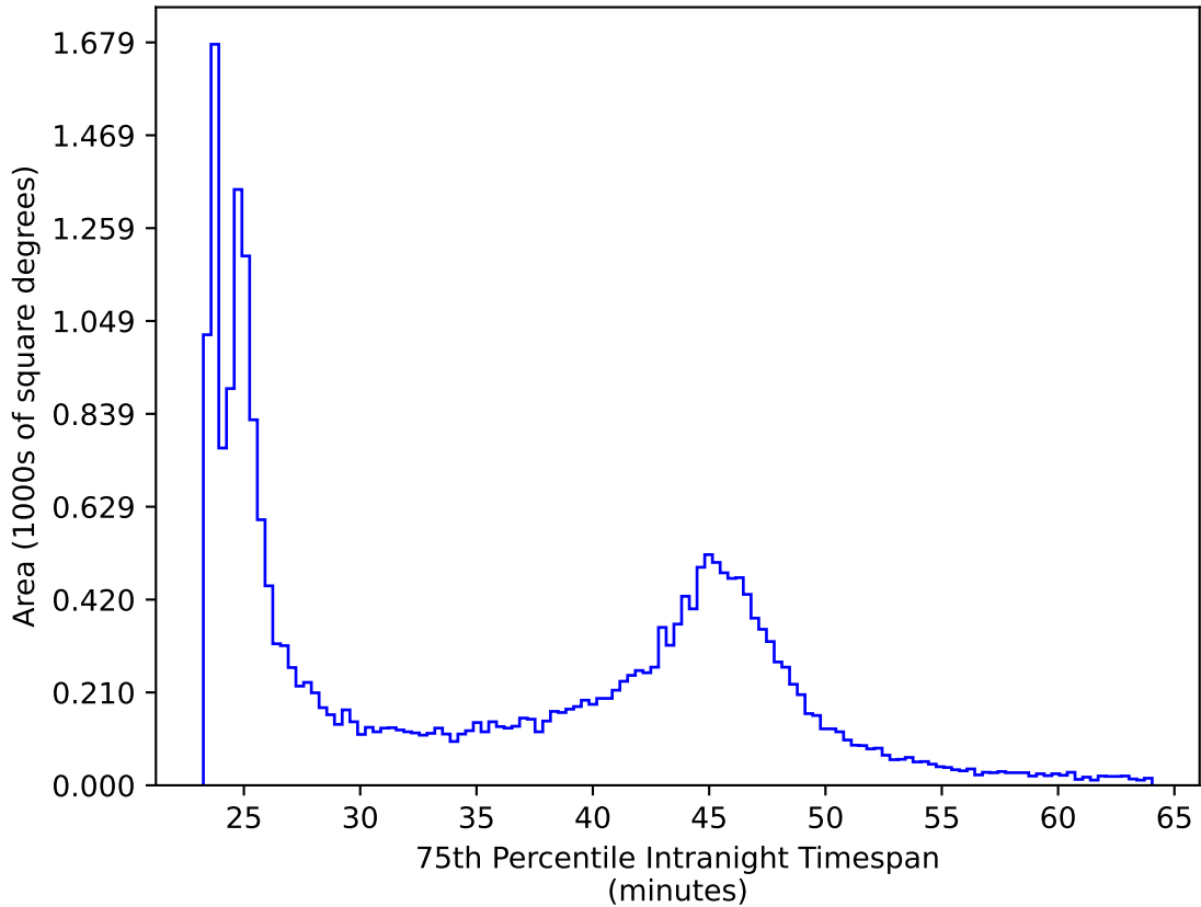
retro_baseline_v2.0_10yrs All sky iz bands: 75th Percentile Intranight Timespan
