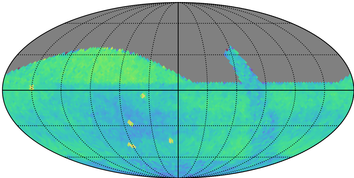
retro_baseline_v2.0_10yrs (g or r or i): PairFraction
