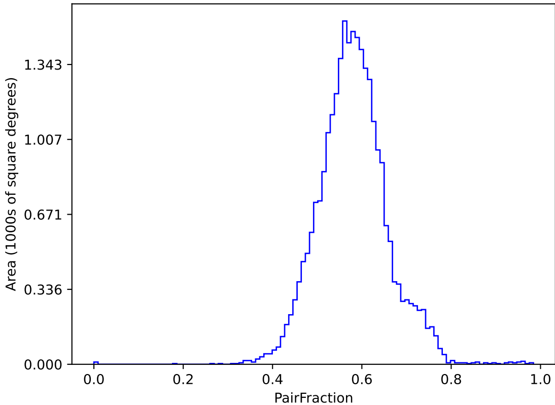
retro_baseline_v2.0_10yrs (g or r or i): PairFraction
