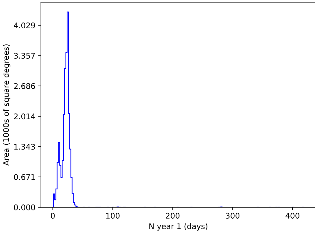
retro_baseline_v2.0_10yrs y and night &lt; 365: N year 1
