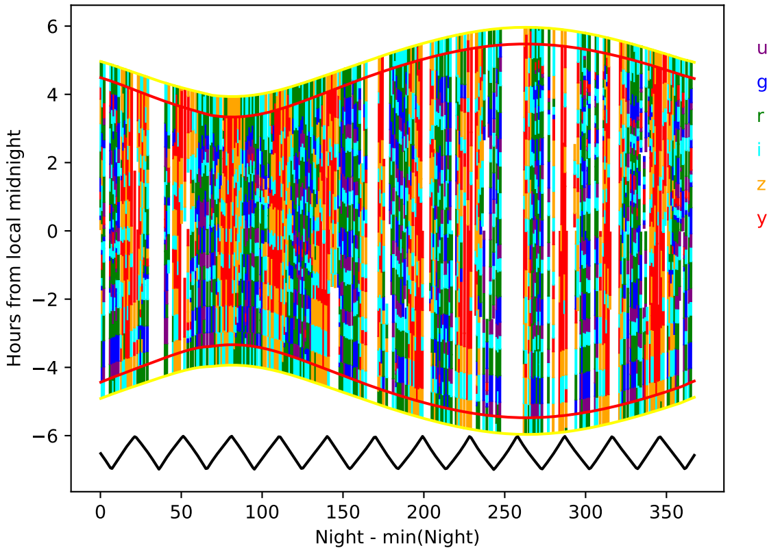
retro_baseline_v2.0_10yrs year 7-8: Hourglass
