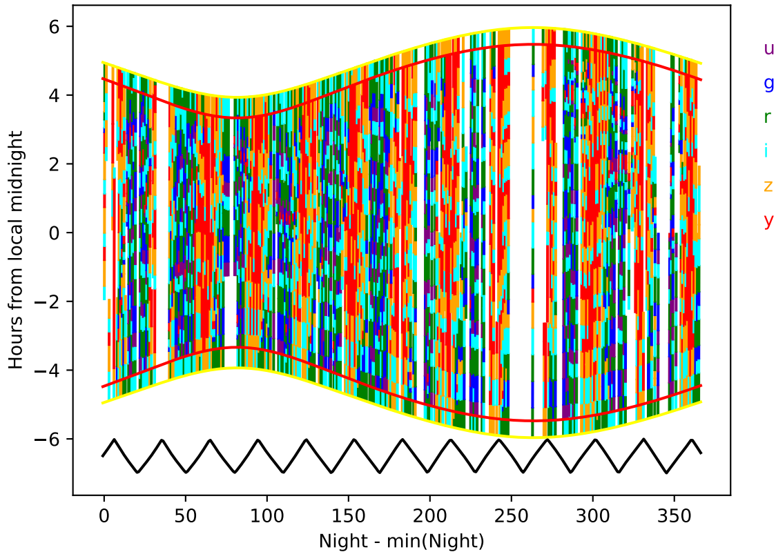
retro_baseline_v2.0_10yrs year 3-4: Hourglass
