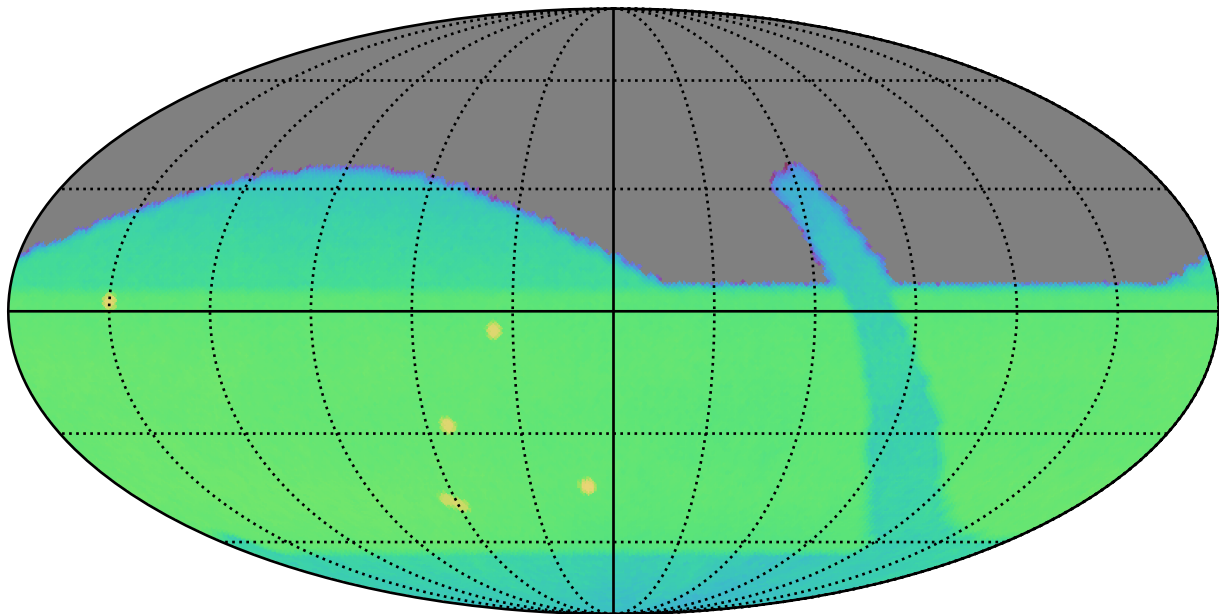
retro_baseline_v2.0_10yrs z: CoaddM5
