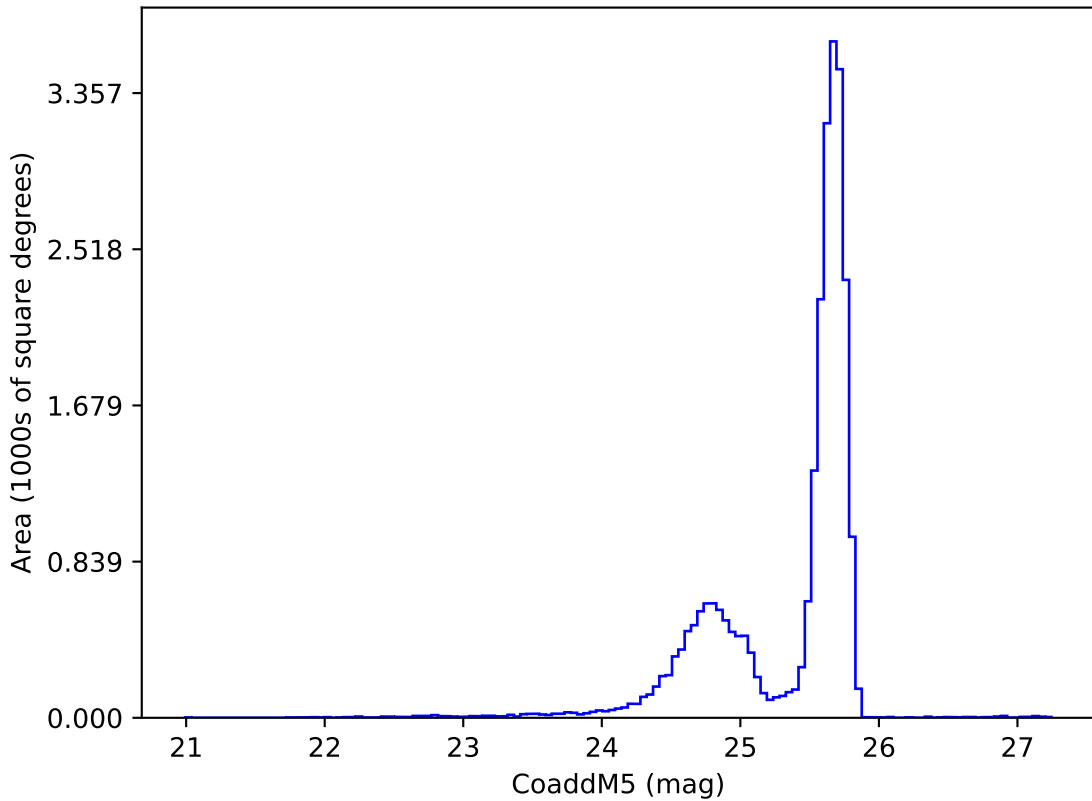
retro_baseline_v2.0_10yrs z: CoaddM5
